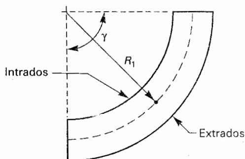
Fig. 304.2.1 Nomenclature for Pipe Bends
