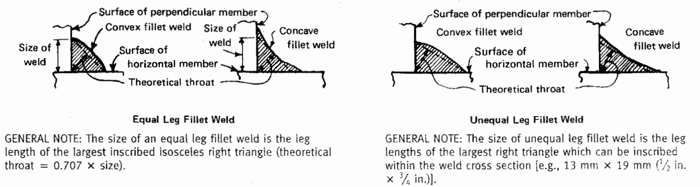
Fig. 328.5.2A Fillet Weld Size
