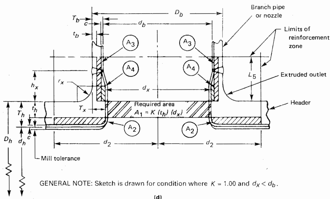
Fig. 304.3.4 Extruded Outlet Header Nomenclature (Cont'd)
